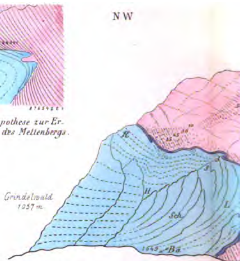
Fig. 4. Der von Gneiss überlagerte Oberjura - Kalkkeil. B - Brunnhorn, Ba - Bäregg beim unteren Eumser, H - Hoch, L - Langenjahn, O - Obere Säggi, R - Raisson, S - Schneider, qt - Eine Quarzbank im Gneiss. Die Ent
